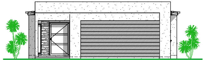
ELEVATION - V2
