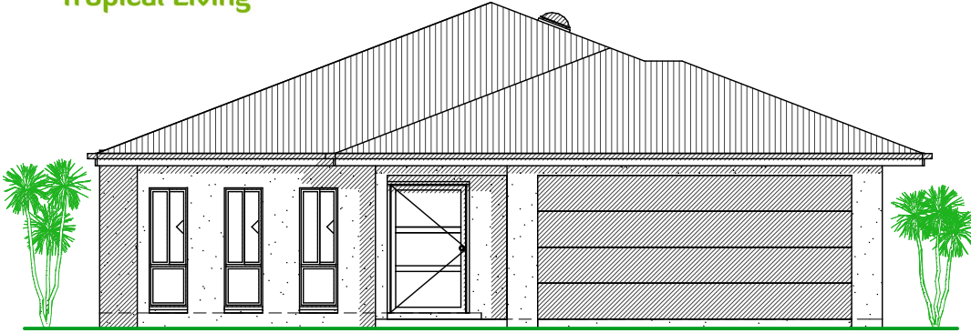
ELEVATION - V1
