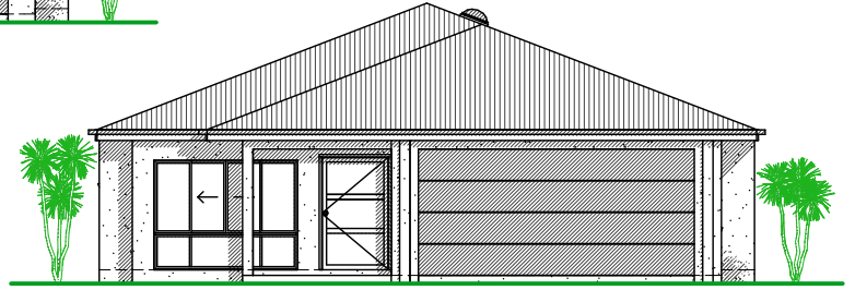
ELEVATION - V2
